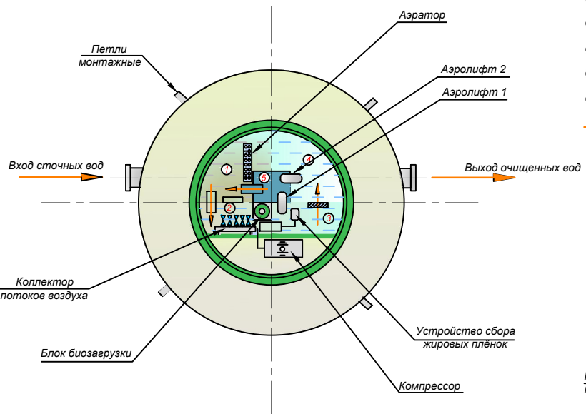
Г(1:5)
